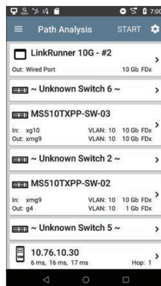
パス解析
