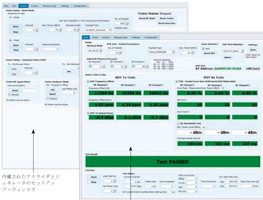
設定とRF測定を実行するメイン・ウィンドウ
